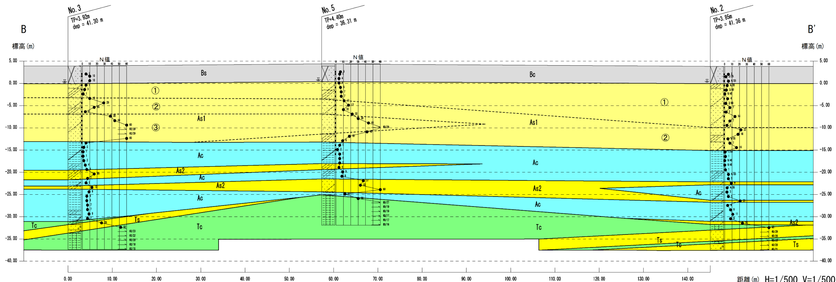
圖 2-4 地質断面圖 (A—A' B—B' 断面)
